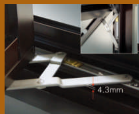
不鏽鋼四連桿加厚設計
