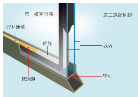
複層玻璃結構
