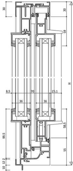
RC框型 YRB-A70 / 單拉窗B型 / 36mm溝寬
