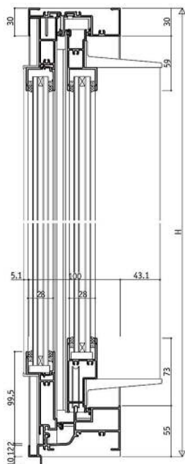
RC框型 YRB-A100 / 雙橫拉真固定D型 / 28mm溝寬
