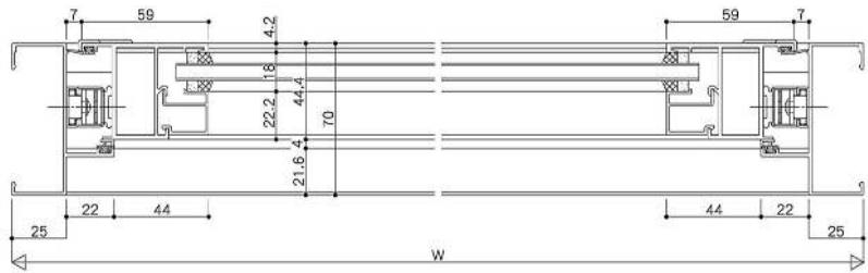
RC框型 YRB-A70 / 推射窗-單扣點式 / 22、28mm溝寬
