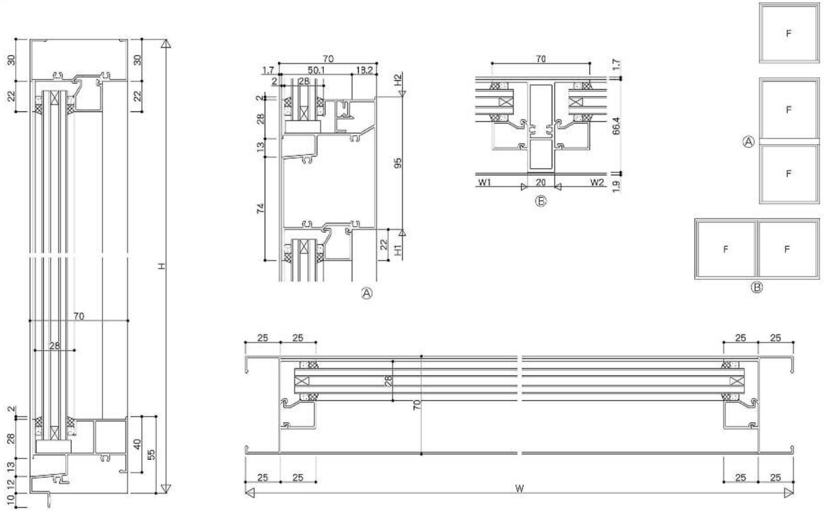
RC框型 YRB-A70/固定窗/28mm溝寬
