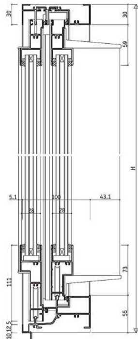
RC框型 YRB-A100/4扇橫拉窗D型/28mm溝寬
