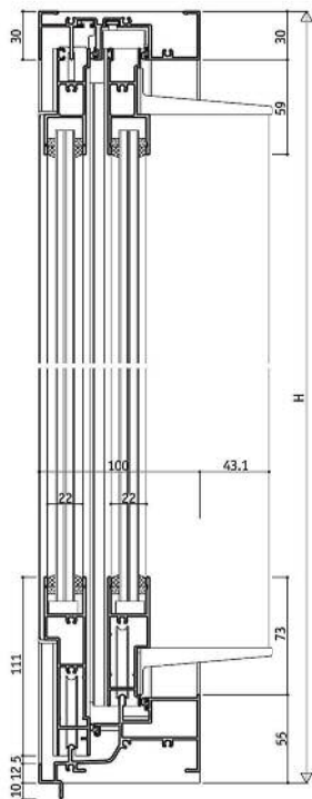
RC框型 YRB-A100/4扇橫拉窗D型/22mm溝寬
