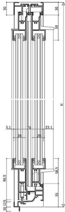
RC框型 YRB-A100/4扇橫拉窗D型/28mm溝寬
