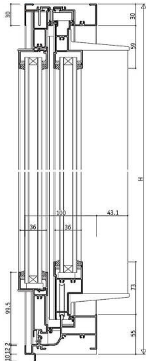
RC框型 YRB-A100 / 雙橫拉真固定D型 / 36mm溝寬
