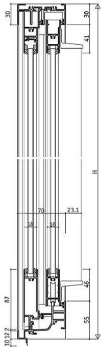
RC框型 YRB-A100 / 雙橫拉真固定D型 / 16mm溝寬
