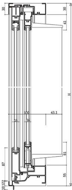
RC框型 YRB-A100 / 雙橫拉真固定D型 / 16mm溝寬
