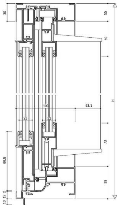
RC框型 YRB-A100 / 單拉窗D型 / 22mm溝寬
