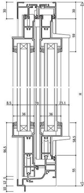
RC框型 YRB-A100 / 2扇横拉窗D型 / 36mm溝寬
