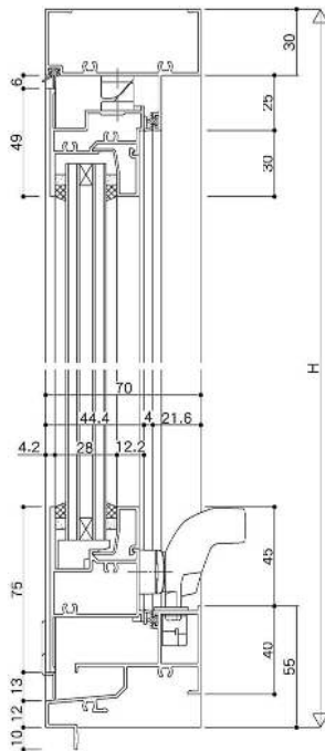
RC框型 YRB-A70 / 推射窗-單扣點式 / 22、28mm溝寬
