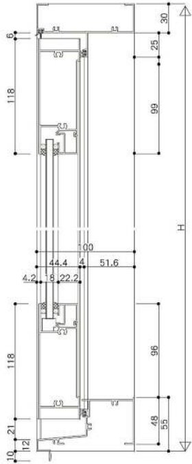
RC框型 YRB-A100 / 氣密門 / 22、28mm溝寬
