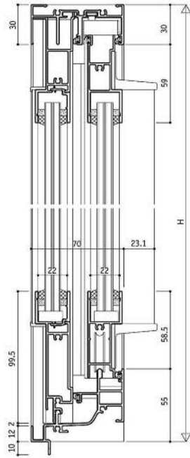
RC框型 YRB-A100 / 單拉窗D型 / 22mm溝寬
