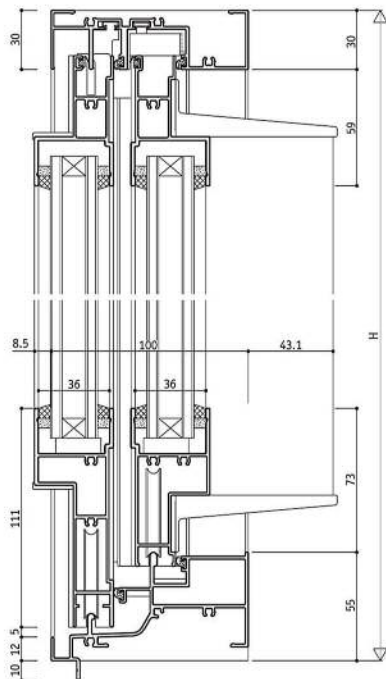
RC框型 YRB-A100 / 2扇横拉窗D型 / 36mm溝寬
