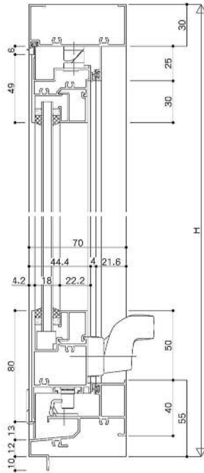
RC框型 YRB-A70 / 推射窗-連動扣點式 / 22、28mm溝寬.....
