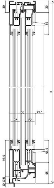
RC框型 YRB-A70/4扇橫拉窗B型/22mm溝寬
