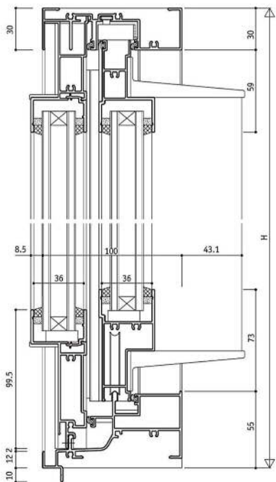
RC框型 YRB-A100 / 單拉窗D型 / 36mm溝寬
