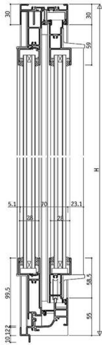
RC框型 YRB-A100 / 雙橫拉真固定D型 / 28mm溝寬
