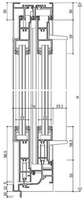
RC框型 YRB-A100/2扇橫拉窗D型/22mm溝寬
