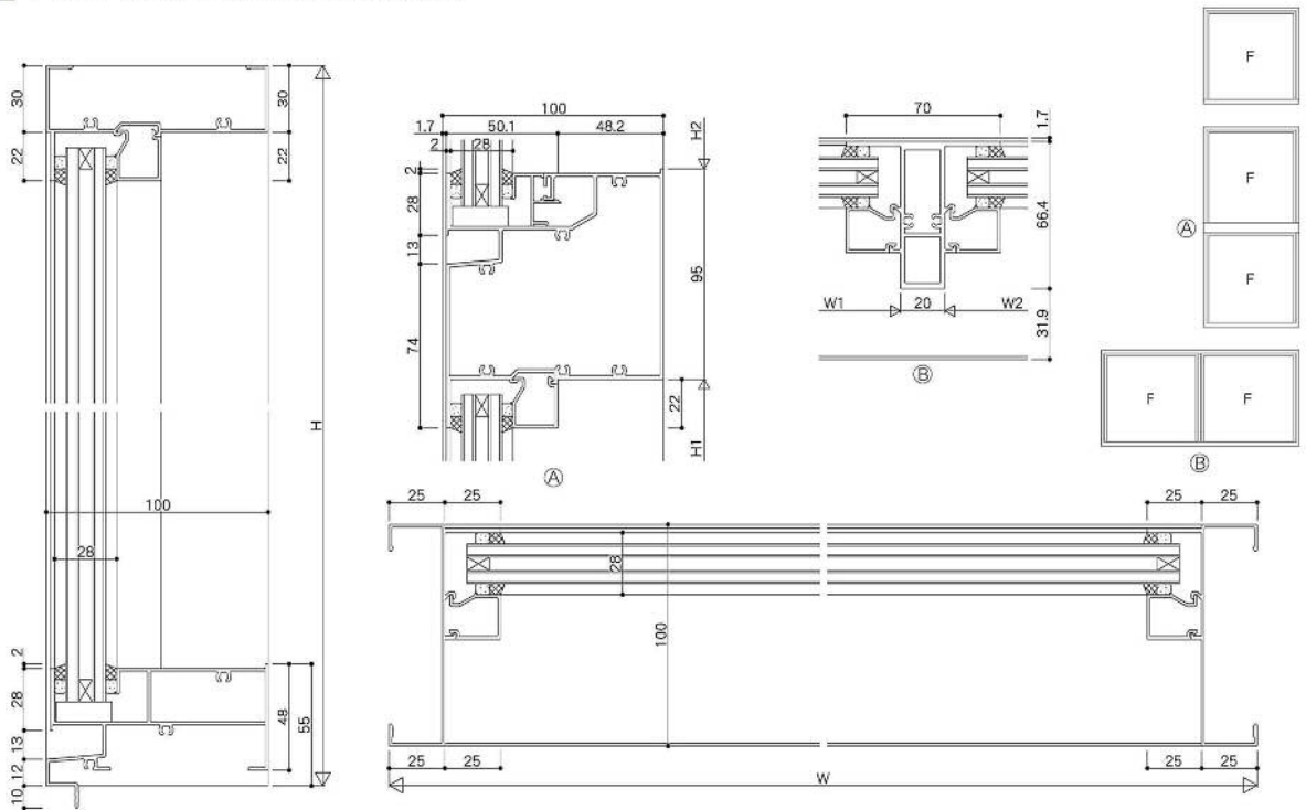
RC框型 YRB-A100/固定窗/28mm溝寬
