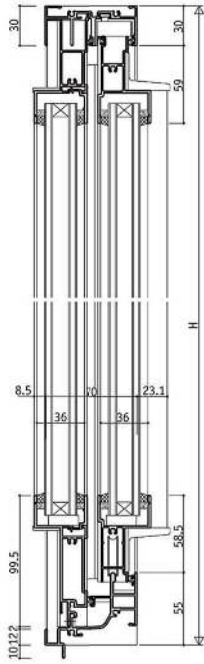
RC框型 YRB-A100 / 雙橫拉真固定D型 / 36mm溝寬
