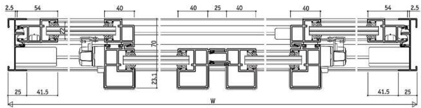
RC框型 YRB-A100/4扇橫拉窗D型/22mm溝寬
