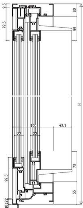
RC框型 YRB-A100 / 雙橫拉真固定D型 / 22mm溝寬
