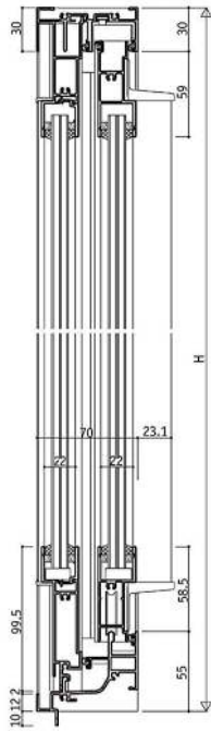
RC框型 YRB-A100 / 雙橫拉真固定D型 / 22mm溝寬
