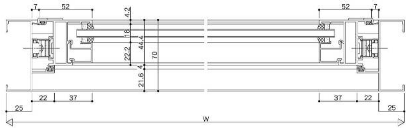
RC框型 YRB-A70 / 推射窗-連動扣點式 / 22、28mm溝寬.....
