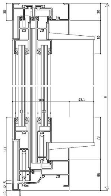
RC框型 YRB-A100/2扇橫拉窗D型/22mm溝寬
