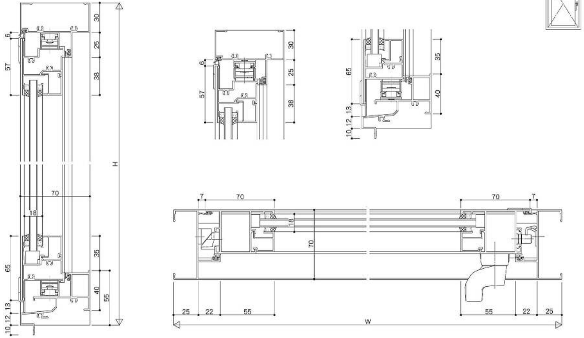
RC框型 YRB-A70 / 推開窗-連動扣點式 / 22、28mm溝寬
