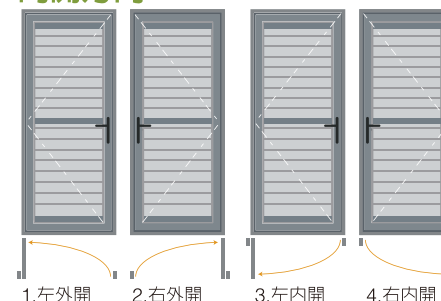
1.左外開 2.右外開 3.左內開 4.右內開
